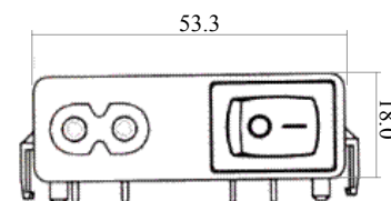
Serie 0721-S: dimensioni
